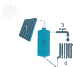
1 zonnecollector 2 opslagvat 3 warm water aansluiting 4 ruimteverwarming 5 verwarmingsinstallatie
