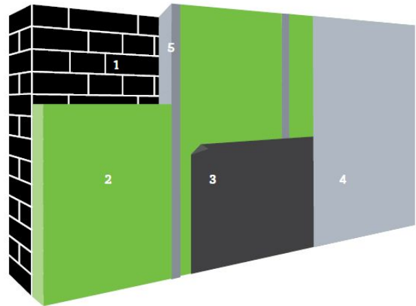
1. Buitengevel | 2. Isolatie | 3. Dampscherp | 4. Binnenafwerking | 5. Stijl- en regelwerk (optioneel)
