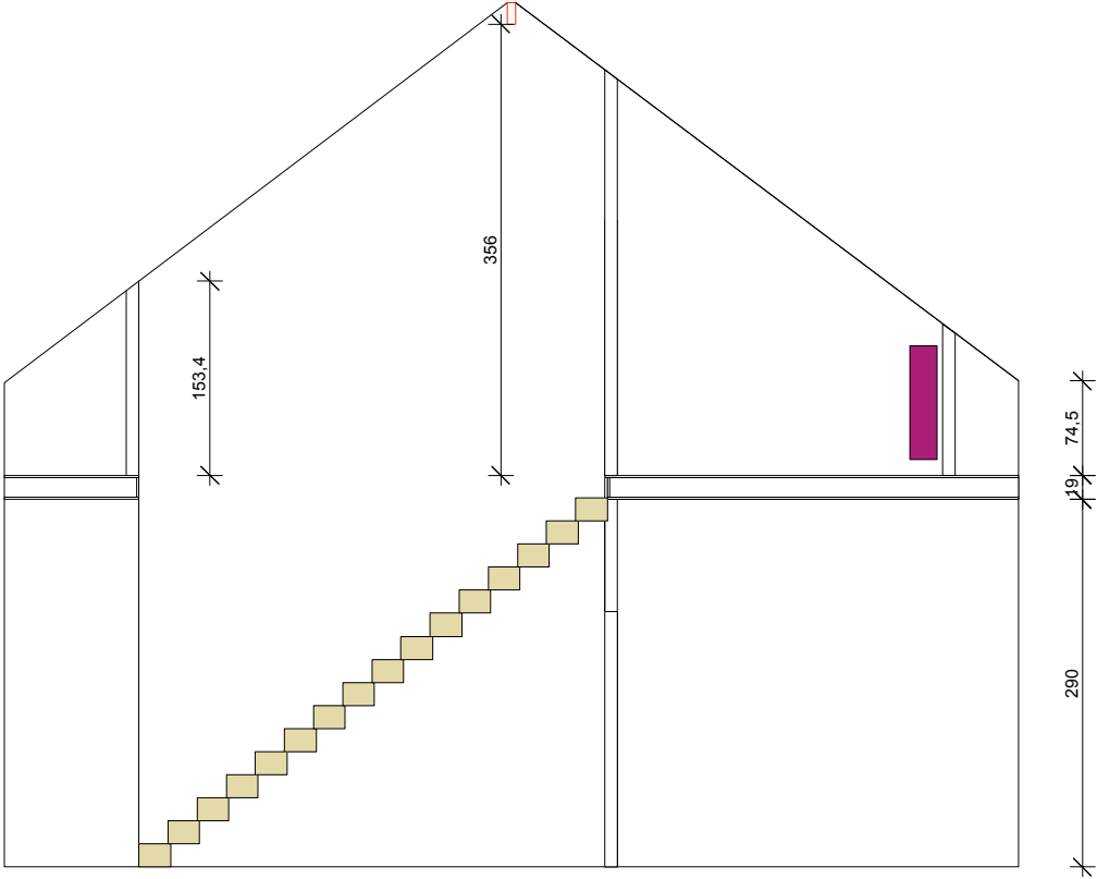
Doorsnede AA'
