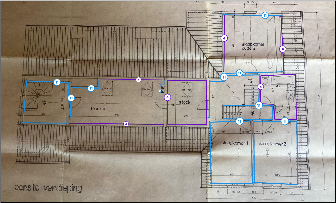
Legende van plan 1.4: Grondplan verdieping
